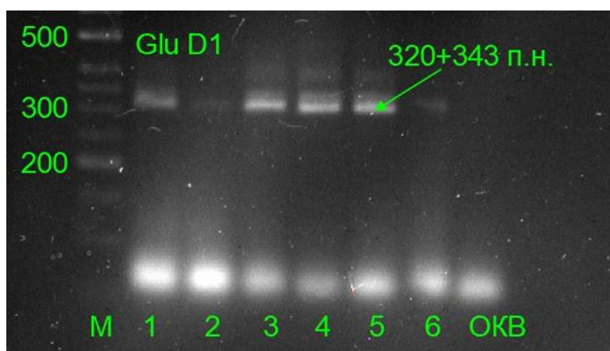
Рисунок 2 - Определение аллелей гена Glu D1 у сортообразцов озимой мягкой пшеницы с маркерами Dx 5F/ DxR, М – маркер молекулярного веса (М) 50 bp; ОКВ - H 2 O деионизированная
